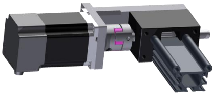
Motormontage 0 Grad, Antriebszapfen rechts MONT003R000
