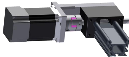
Motormontage 90 Grad, Antriebszapfen rechts MONT003R090
