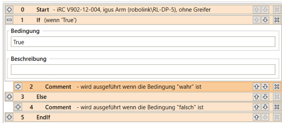
Abbildung 16: Die If-Anweisung verzweigt den Programmfluss.
