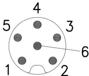
Abbildung 24: Belegung der DIO-Buchse am Arm
