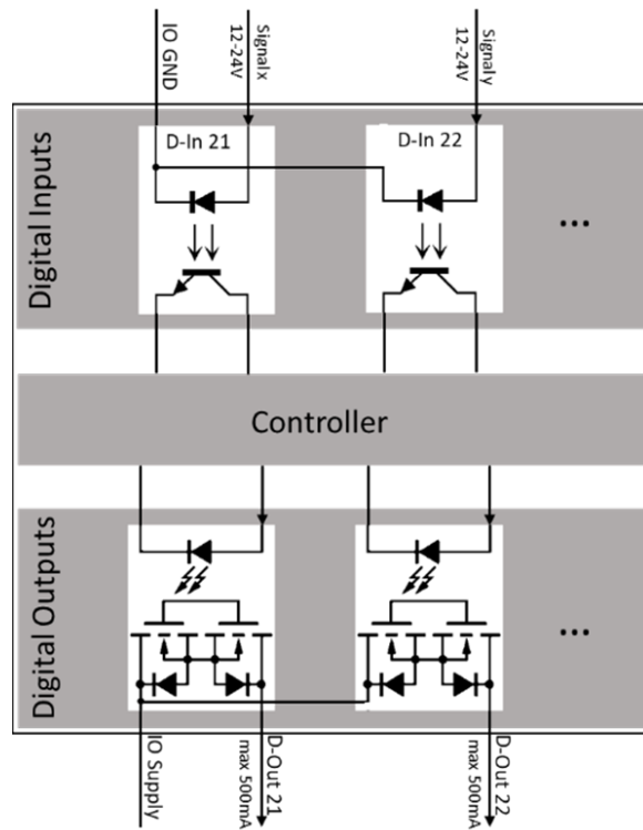
Abbildung 25: Interner Aufbau eines DIO-Moduls
