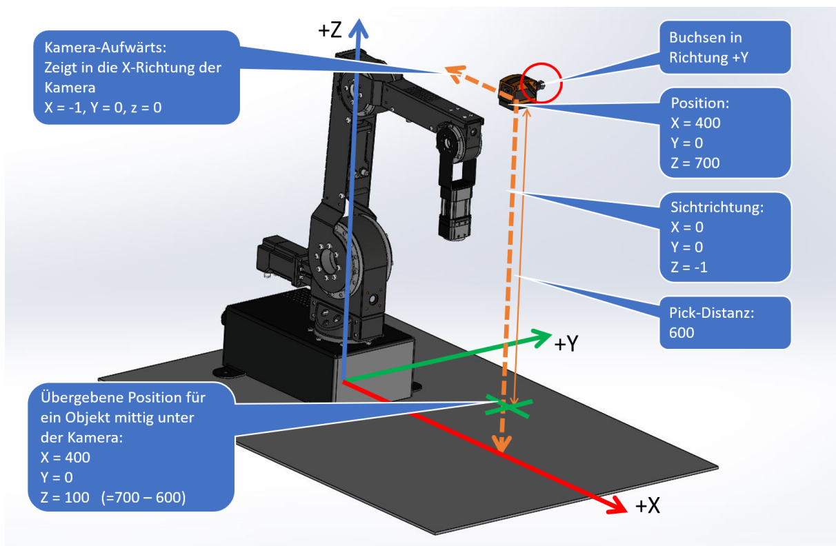
Abbildung 27: Vermessung der Kameraposition und -ausrichtung.
